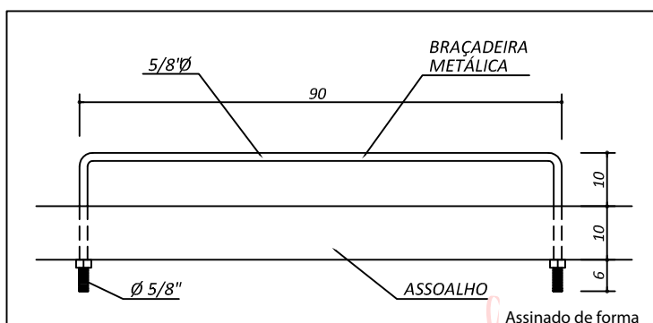
Detalhe 03 Det. de braçadeira metálica do rodeiro Sem Escala
